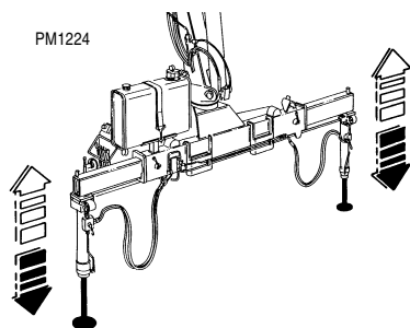
COMANDO SFILO MARTINETTI STABILIZZATORI OUTRIGGER CYLINDER EXTENSION CONTROL
